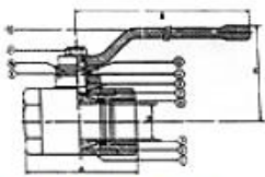
3. Шаровой кран Три раунда Pc орган Полный Диаметр болта до 70 бар
