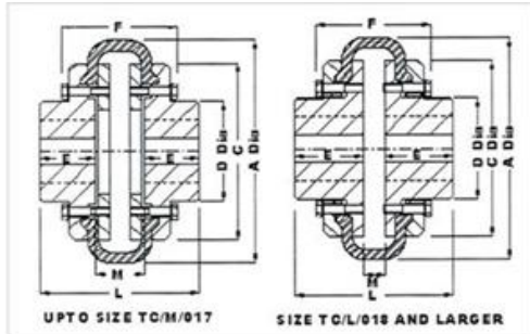
热电偶橡胶轮胎联轴器
