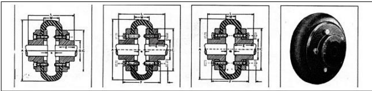
F轮胎联轴器
