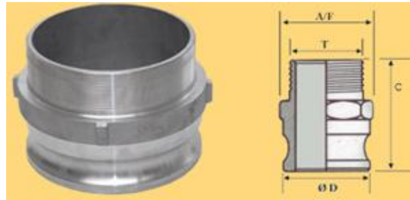
Camlock男适配器F
